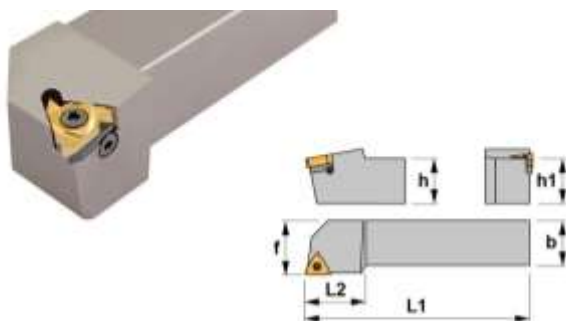
STXNR2020K16
